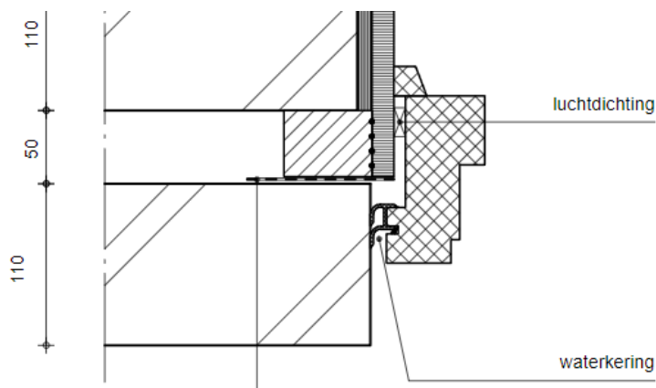
Tekening 11.B4.04
